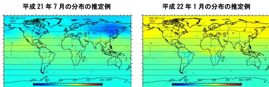
図7 二酸化炭素収支推定結果に基づいて大気輸送モデルを用いた数値シミュレーション計算から得られる二酸化炭素の濃度分布の推定例。
