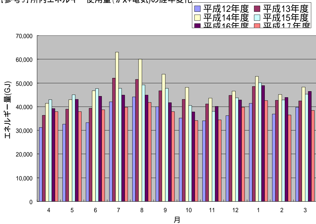
【参考5】所内エネルギー使用量(ガス+電気)の経年変化
